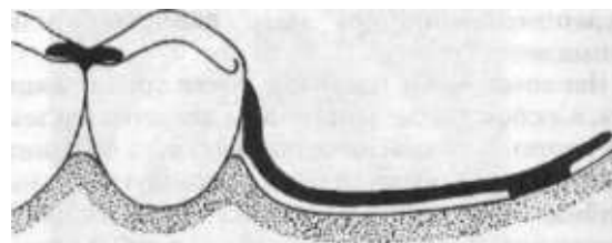
Рис. 406. Предупреждение оседания металлического каркаса при замене воскового базиса на пластмассовый.
