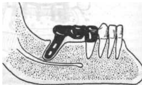
Рис. 344. Мостовидный протез с дистальной опорой на имплантат.
