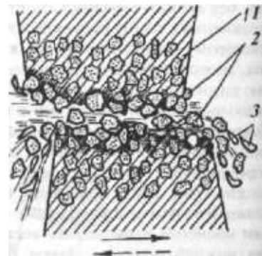
Рис. 560. Зона притирки воскабразивных окклюзионных валиков: 1 — восковая композиция; 2 — абразивные зёрна, 3 — стружка.
