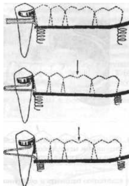
Рис. 400. Принцип действия вертикального дробителя нагрузок.
