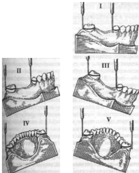
Рис. 416. Положение моделей в параллелометре относительно диагностического стержня.
