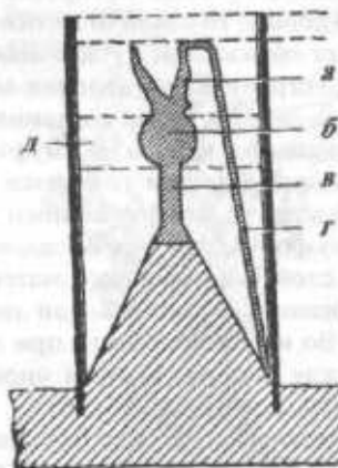
Рис. 289. Схема литейной кюветы в разрезе: а — восковая модель; б — противоусадочная муфта; в — литейный канал; г — канал для отвода воздуха из литейной формы; д — тепловой центр кюветы.
