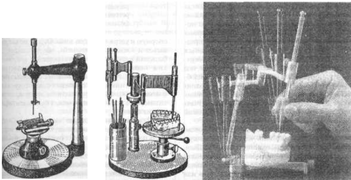
Рис. 412. Различные типы параллелометров.
