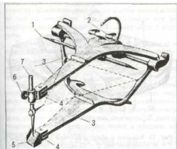
Рис. 49. Средний анатомический артикулятор. 1 — горизонтальный стержень; 2 — пружины; 3 — верхняя и нижняя пластины, 4 — соединительные муфты; 5 — резцовая площадка; 6 — муфта с винтом, удерживающим стрелку — указатель центра; 7 — вертикальный штифт.
