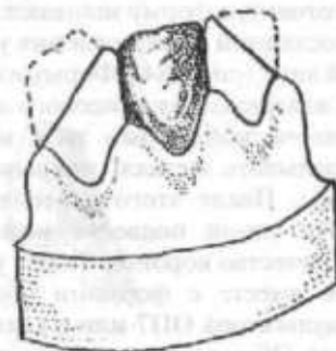
Рис. 187. Фрагмент гипсовой модели с восковой репродукцией пластмассовой коронки, подготовленный для гипсовки в кювете. Крайние зубы с внешних сторон конусообразно срезают.
