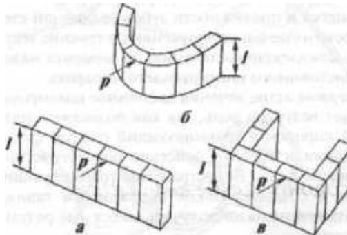
Рис. 463. Распределение шинирующих блоков. а — линейное; б — по дуге; в — в виде буквы /; / — высота блока.
