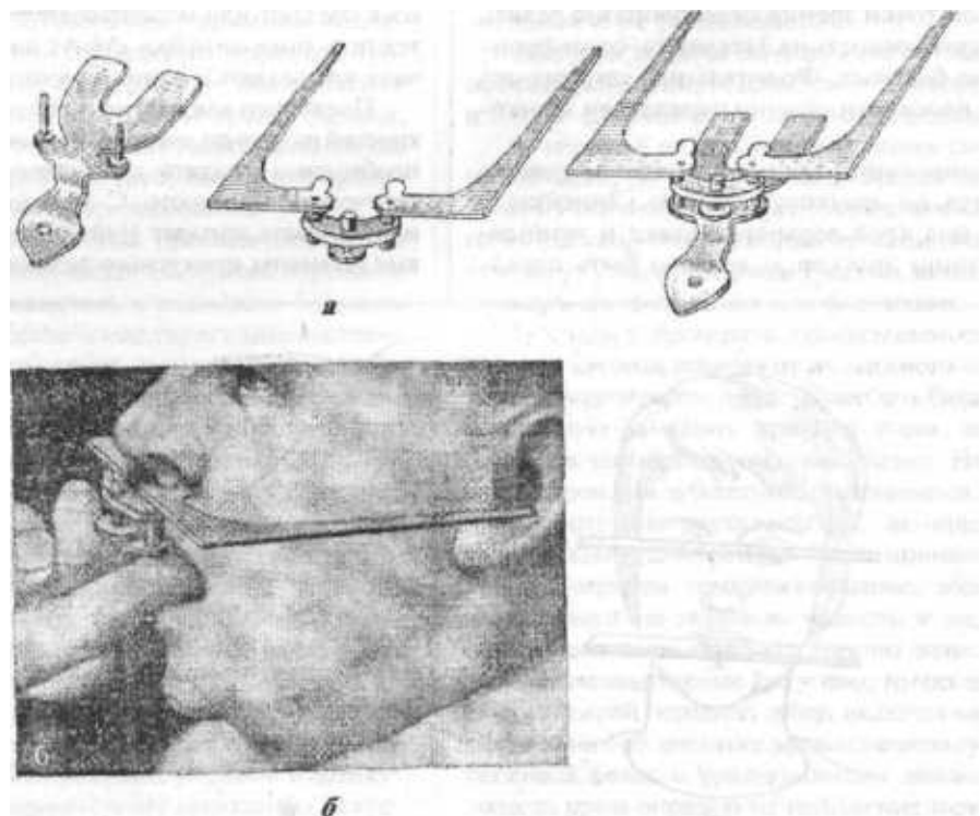
Рис. 535. Аппарат Ларина:
