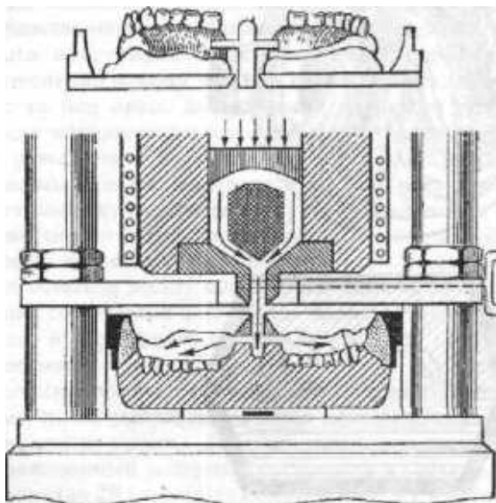
Рис. 375. Схема литевой формы для изготовления протезов из термопластических масс.
