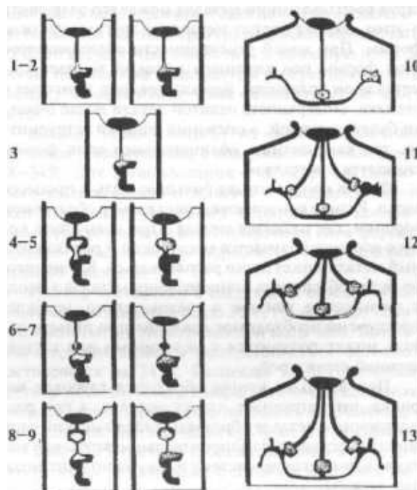
Рис. 286. Образование усадочных раковин и их положение в литниковой системе малых (слева) и больших (справа) по протяженности деталей (объяснение в тексте).
