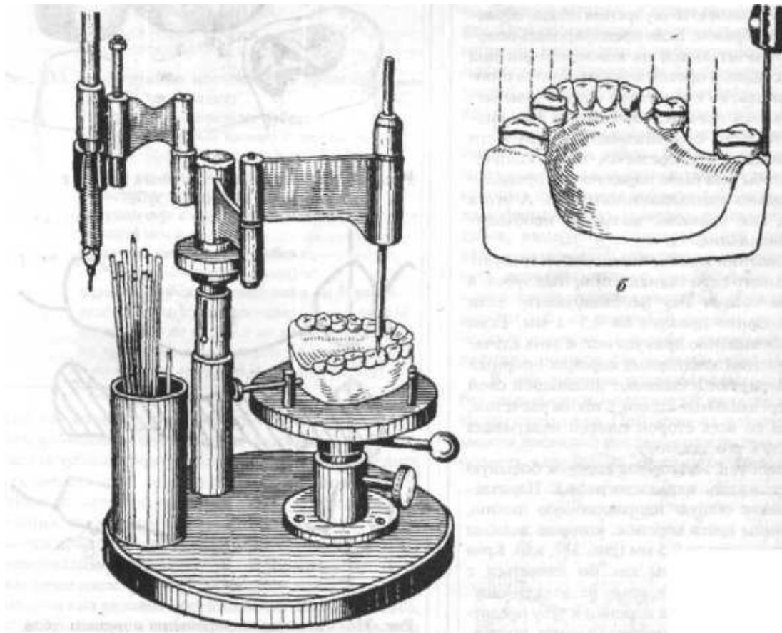
Рис. 317. Параллелограф (а); модель с очерченной направляющей линией (линия обзора), указывающей границы экваторных коронок (б).
