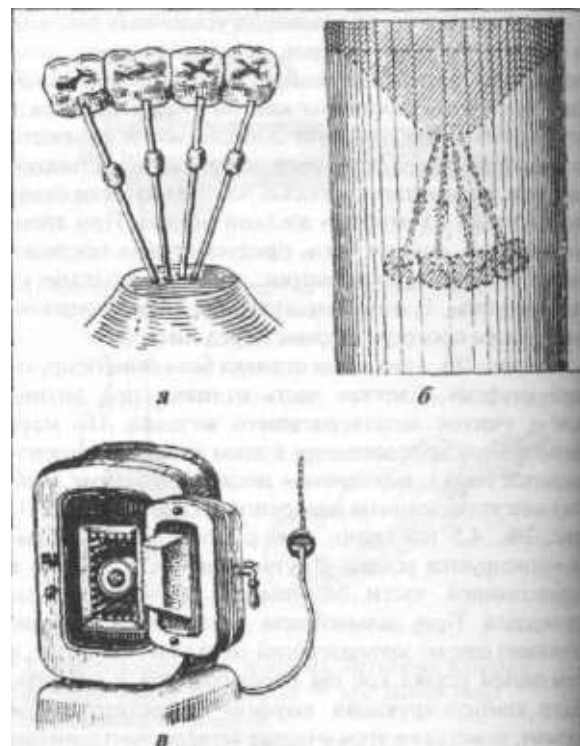
Рис. 288. Замена металлом посковой модели тела протеза: а — укрепление тела протеза на конусе; б — разрез отливочной кюветы, показано расположение в нем тела протеза; в — муфельная печь.
