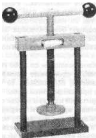
Рис. 373. Пресс для плотного соединения частей кюветы перед полимеризацией.
