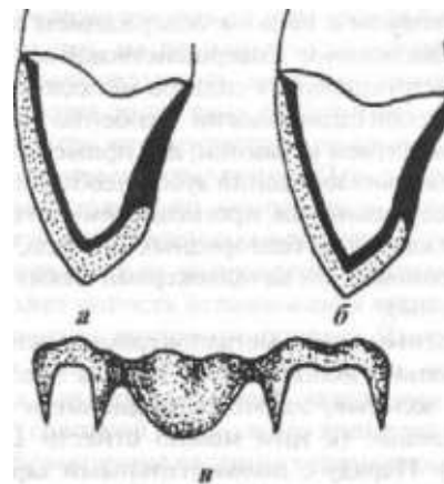
Рис. 303. Особенности моделировки каркаса металлокерамического мостовидного протеза: а —правильная моделировка каркаса опорной коронки с гирляндой; б —неправильная моделировка каркаса опорной коронки (колпачок от моделирован с острым режущим краем, а гирлянда с оральной стороны в месте перехода в колпачок имеет поднутрение); в —каркас мостовидного протеза с плавными переходами опорных коронок в промежуточную часть.
