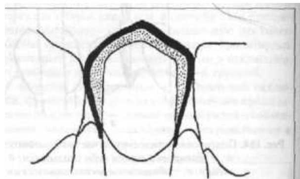
Рис. 167. Моделировка штампованной коронки. На культе препарированного зуба из гипса показан слой воска (точечная штриховка), уменьшенный в объеме по сравнению с размерами естественного зуба на толщину штампованной коронки (обозначена сплошной линией).
