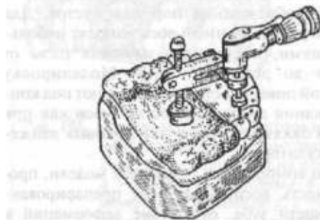
Рис. 194. Внутриротовой параллелометр (изодром).
