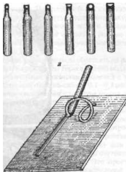
Рис. 425. Ножи для стандартных восковых заготовок: а — формы ножей; б — момент получения воска определенного профиля.
