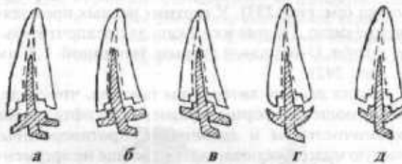
Рис. 244. Варианты подготовки поверхности корня при изготовлении штифтового зуба по Л.В. Ильиной-Маркосин: а, б, в — правильная подготовка; г, д — неправильная.
