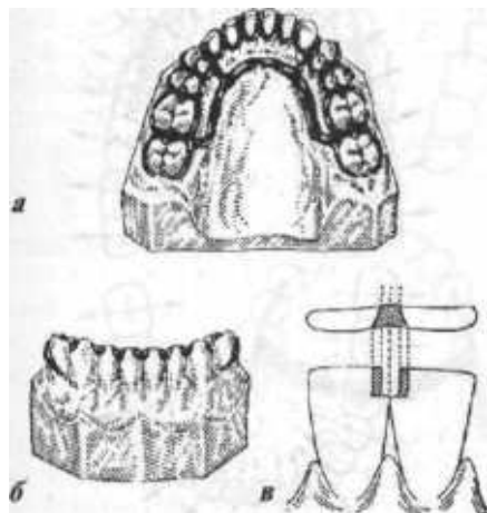
Рис. 477. Съемная цельнолитая шина: а - общий вид; б — вид спереди; в — схема подготовки зубов для когтевидных накладок.
