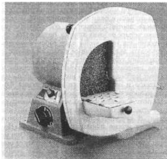
Рис. 410. Специальный шлифмотор с меняющимися дисками и водяным орошением для обрезания гипсовых моделей.
