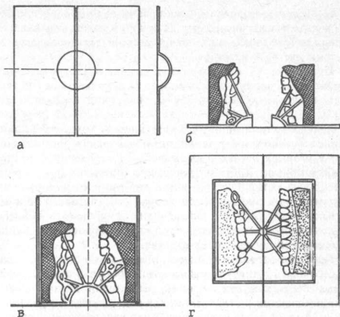
63. Схема формовки (С. Д. Богословский):
