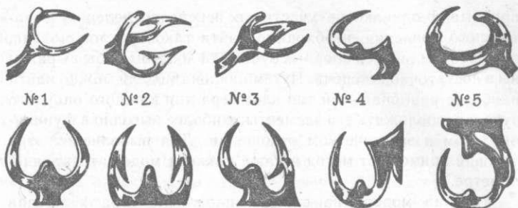
58. Виды литых опорно-удерживающих кламмеров системы Ней.
